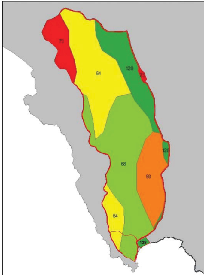
Figura 4 – Carta litologica
